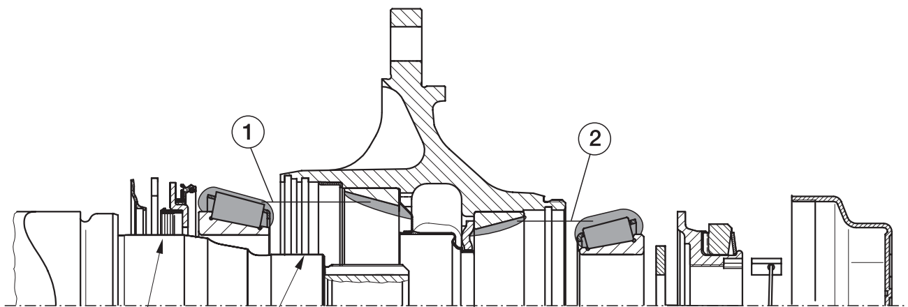
Lagersitze des Achsschenkels mit BPW ECO Assembly and Protection Spray einsprühen Spray the bearing seats of the axle stub with BPW ECO Assembly and Protection Spray Lubrifier les logements des roulements de fusée avec le spray BPW ECO Assembly and Protection
